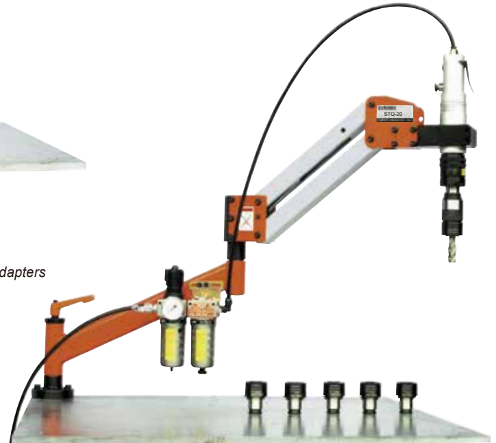
STQ-20 M3~M20 STQ-22 M3~M22 STQ-24 M3~M24 STQ-27 M3~M27 Air Tapping Machine
