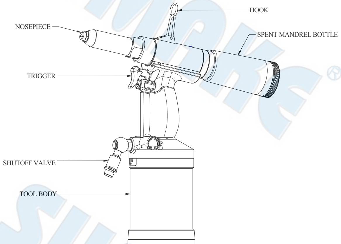
Fig. 1 ST-66155V Rivet-Pull Tool
